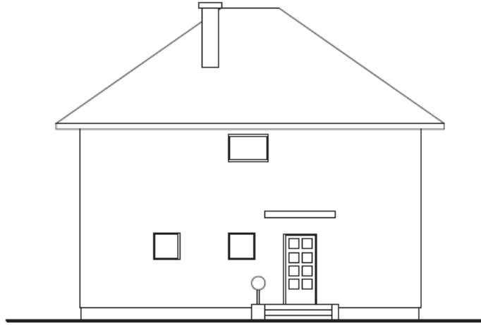
PROČELJE JUG
